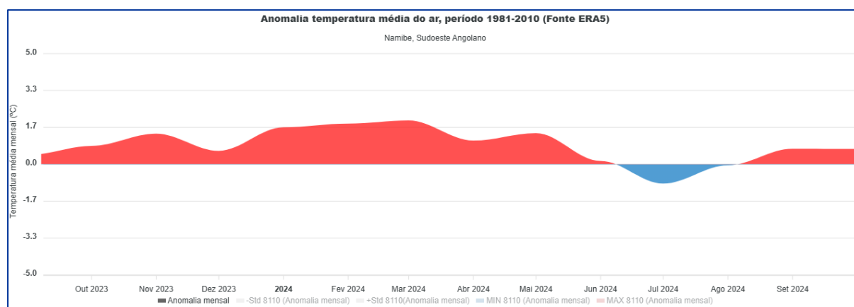
FIGURA 3-3. GRÁFICO DAS ANOMALIAS DE TEMPERATURA DO AR A 2M, NA PROVÍNCIA DO NAMIBE, AO LONGO DA ÉPOCA DAS CHUVAS 2023/24.
