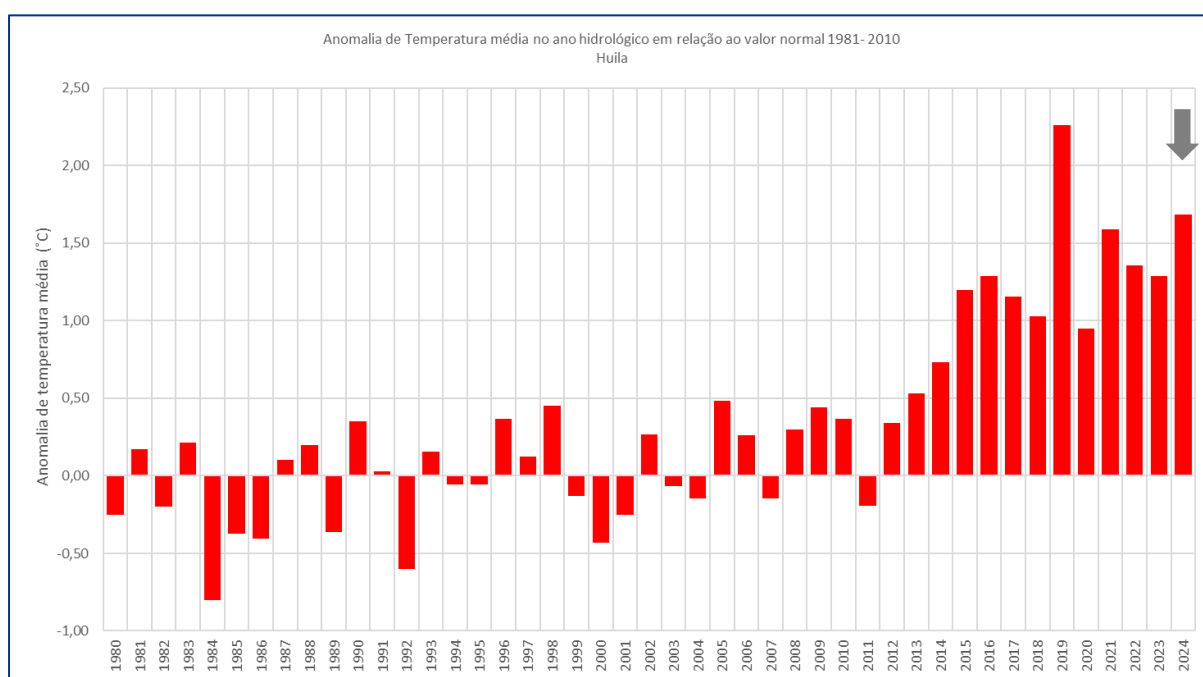
FIGURA 2-2 – GRÁFICO DAS ANOMALIAS DE TEMPERATURA DO AR A 2M, NA PROVÍNCIA DA HUÍLA, EM CADA ANO HIDROLÓGICO DESDE 1979.
