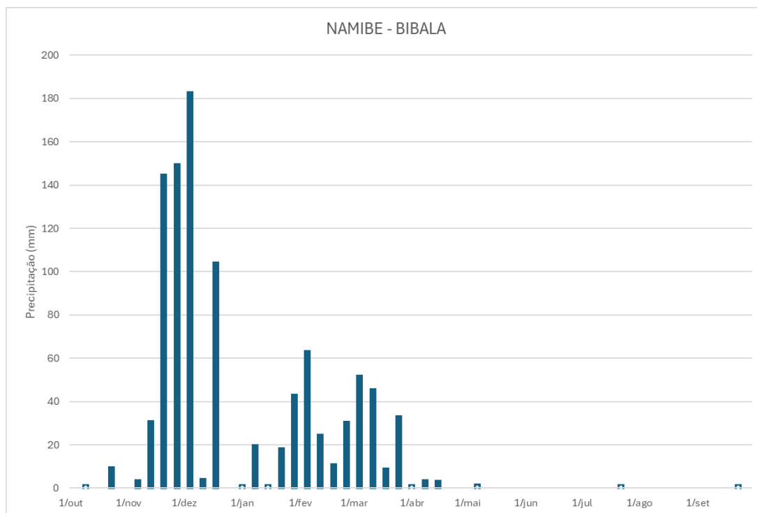
FIGURA 5-2. ACUMULADOS SEMANAIS DE PRECIPITAÇÃO, AO LONGO DO ANO HIDROLÓGICO 23/24, NA ESTAÇÃO FRESAN DE BIBALA
