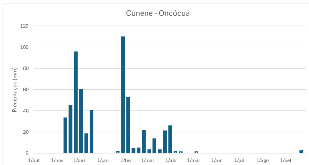
FIGURA 5-3. ACUMULADOS SEMANAIS DE PRECIPITAÇÃO, AO LONGO DO ANO HIDROLÓGICO 23/24, NA ESTAÇÃO FRESAN DE ONCÓCUA
