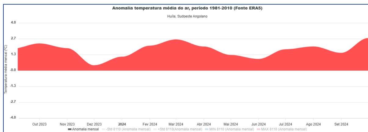
FIGURA 2-3 - GRÁFICO DAS ANOMALIAS DE TEMPERATURA DO AR A 2M, NA PROVÍNCIA DA HUÍLA, AO LONGO DO ANO HIDROLÓGICO 23/24.
