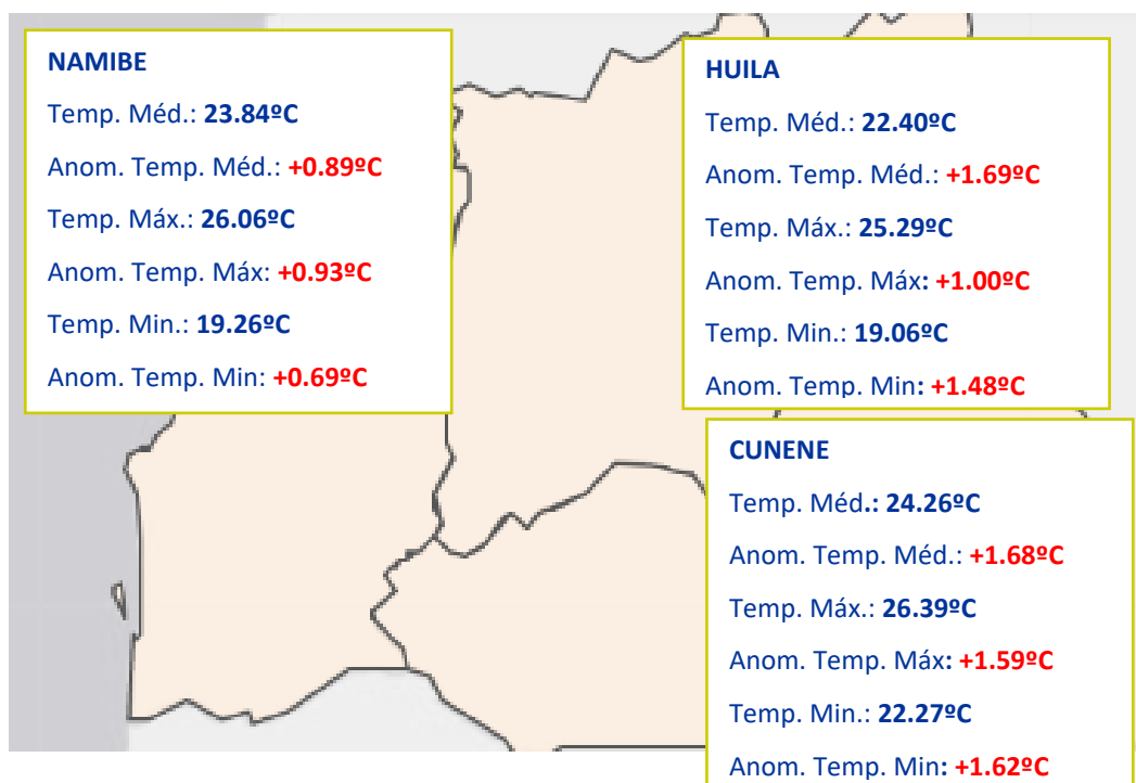
FIGURA 1-2: MAPA DOS VALORES DE TEMPERATURA E ANOMALIA, EM RELAÇÃO AO NORMAL (81-2010), PARA AS 3 PROVÍNCIAS DO SW ANGOLANO, DURANTE O ANO HIDROLÓGICO 23/24.
