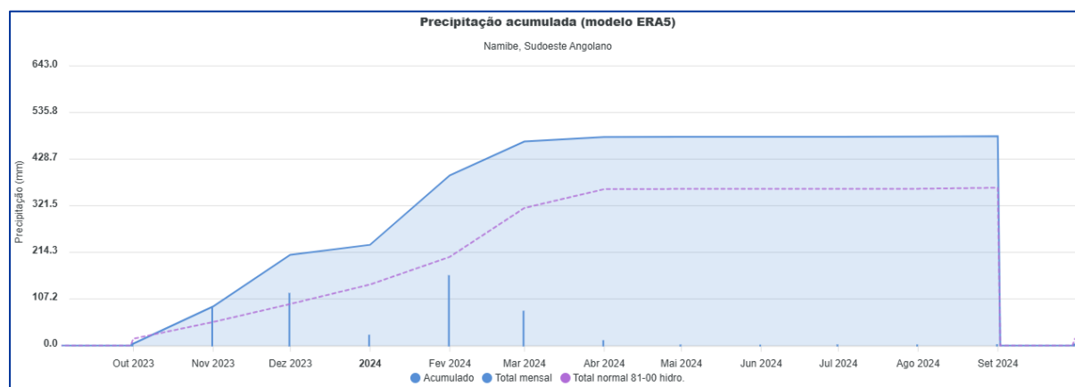
FIGURA 3-1. GRÁFICO DA PRECIPITAÇÃO ACUMULADA AO LONGO DA ÉPOCA DAS CHUVAS 2023/24 NA PROVÍNCIA DO NAMIBE. OS VALORES NORMAIS CORRESPONDEM À CLIMATOLOGIA 1981-2010.
