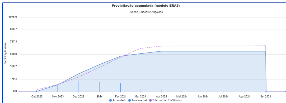
FIGURA 4-1. GRÁFICO DA PRECIPITAÇÃO ACUMULADA AO LONGO DO ANO HIDROLÓGICO 2023/24 NA PROVÍNCIA DO CUNENE. OS VALORES NORMAIS CORRESPONDEM À CLIMATOLOGIA 1981-2010.
