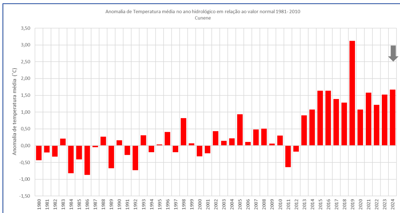
FIGURA 4-2 - GRÁFICO DAS ANOMALIAS DE TEMPERATURA DO AR A 2M, NA PROVÍNCIA DO CUNENE, EM CADA ANO HIDROLÓGICO DESDE 1979.
