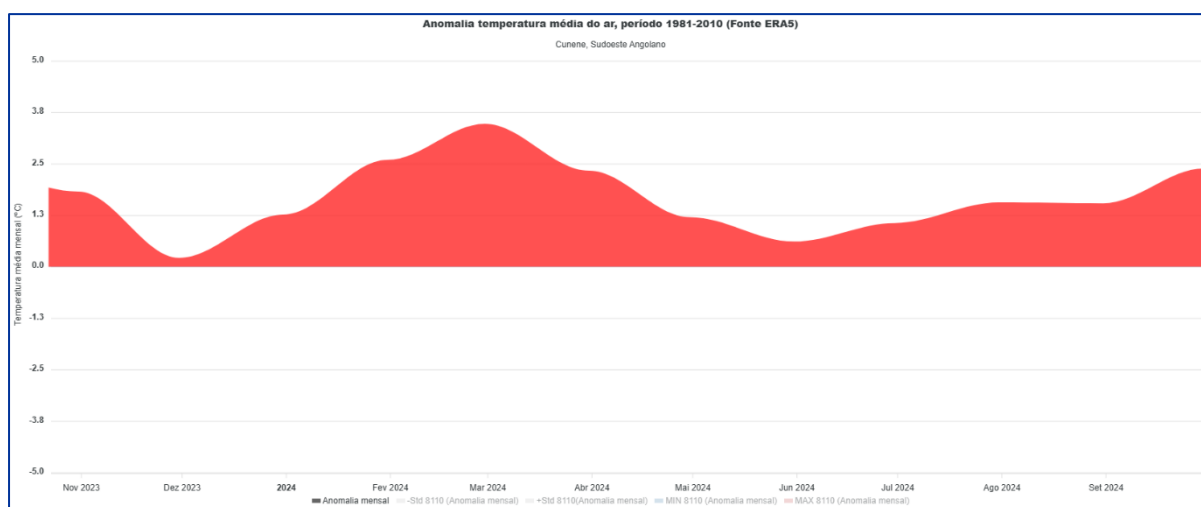
FIGURA 4-3. GRÁFICO DAS ANOMALIAS DE TEMPERATURA DO AR A 2M, NA PROVÍNCIA DO CUNENE, AO LONGO DO ANO HIDROLÓGICO 2023/24.
