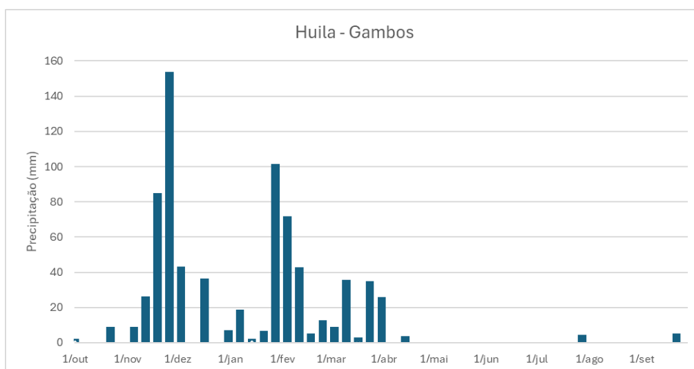
FIGURA 5-1: ACUMULADOS SEMANAIS DE PRECIPITAÇÃO, AO LONGO DO ANO HIDROLÓGICO 23/24, NA ESTAÇÃO FRESAN DE GAMBOS.
