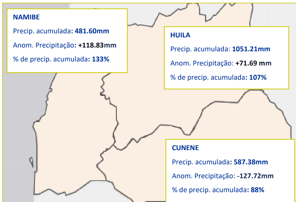
FIGURA 1-1: MAPA DOS VALORES DE ANOMALIA DE PRECIPITAÇÃO E PERCENTAGEM DE PRECIPITAÇÃO EM RELAÇÃO AO NORMAL (81-2010), PARA AS 3 PROVÍNCIAS DO SW ANGOLANO, DURANTE O ANO HIDROLÓGICO 2023/24.
