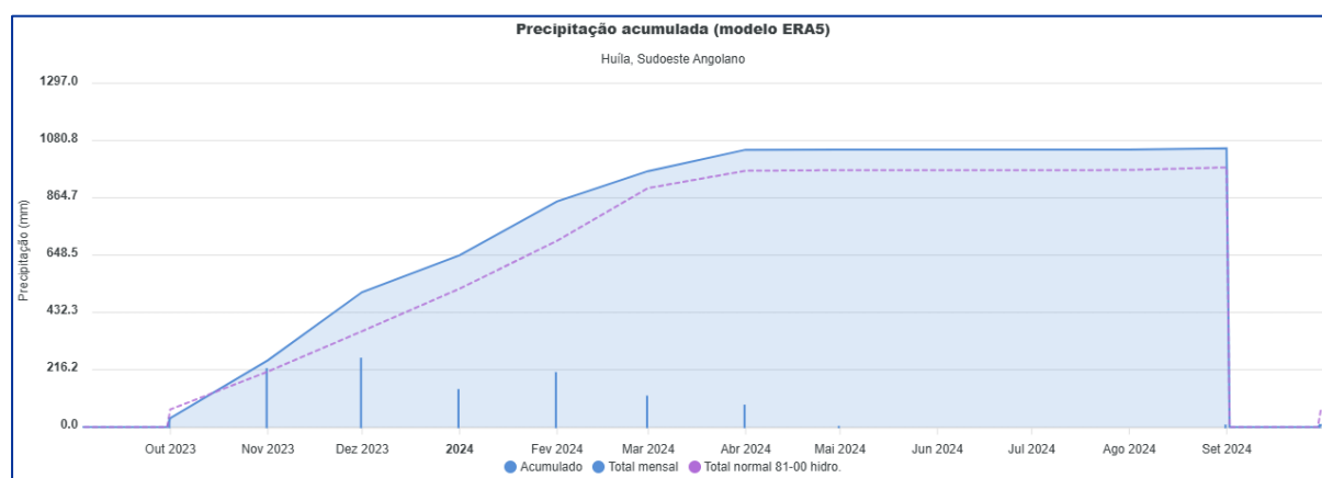
FIGURA 2-1. GRÁFICO DA PRECIPITAÇÃO ACUMULADA AO LONGO DO ANO HIDROLÓGICO 2023/24 NA PROVÍNCIA DA HUÍLA. OS VALORES NORMAIS CORRESPONDEM À CLIMATOLOGIA 1981-2010.
